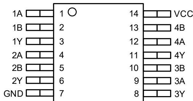
SOP14/TSSOP14
