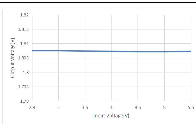
Output Voltage VS Input Voltage(I OUT =10mA)
