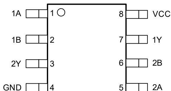
VSSOP8/MSOP8
