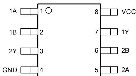
VSSOP8/MSOP8
