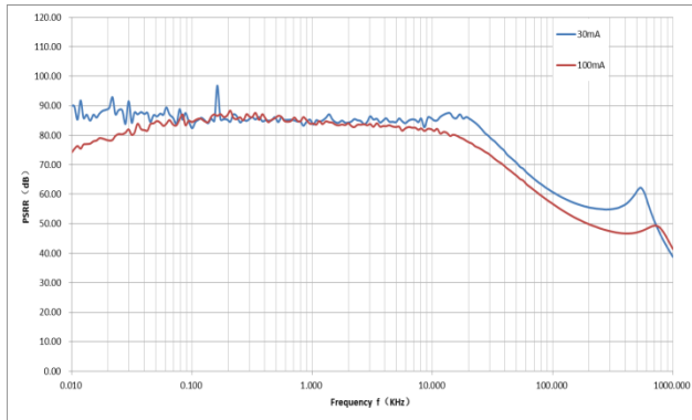
LDO4 PSRR-VIN
