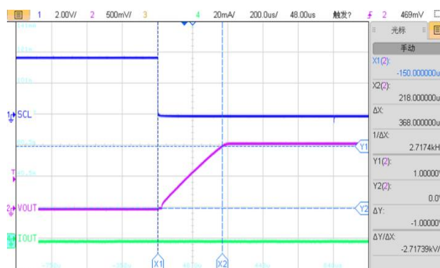
LDO1/2 Ton
