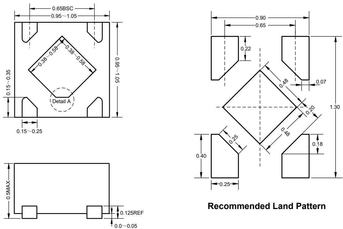
Detail A: (PIN1 shape)
