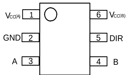
SC70-6
