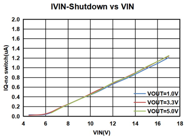
Figure3.IVIN-Shutdown vs VIN
