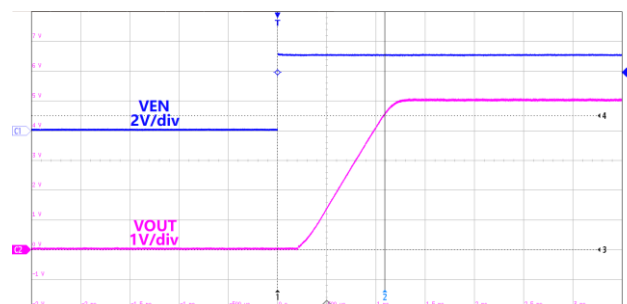
Figure40.Soft Start
