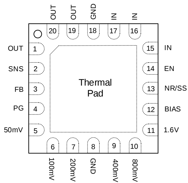
QFN20 (ET5B001YB)
